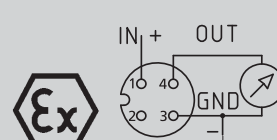
Connecteur M12x1
